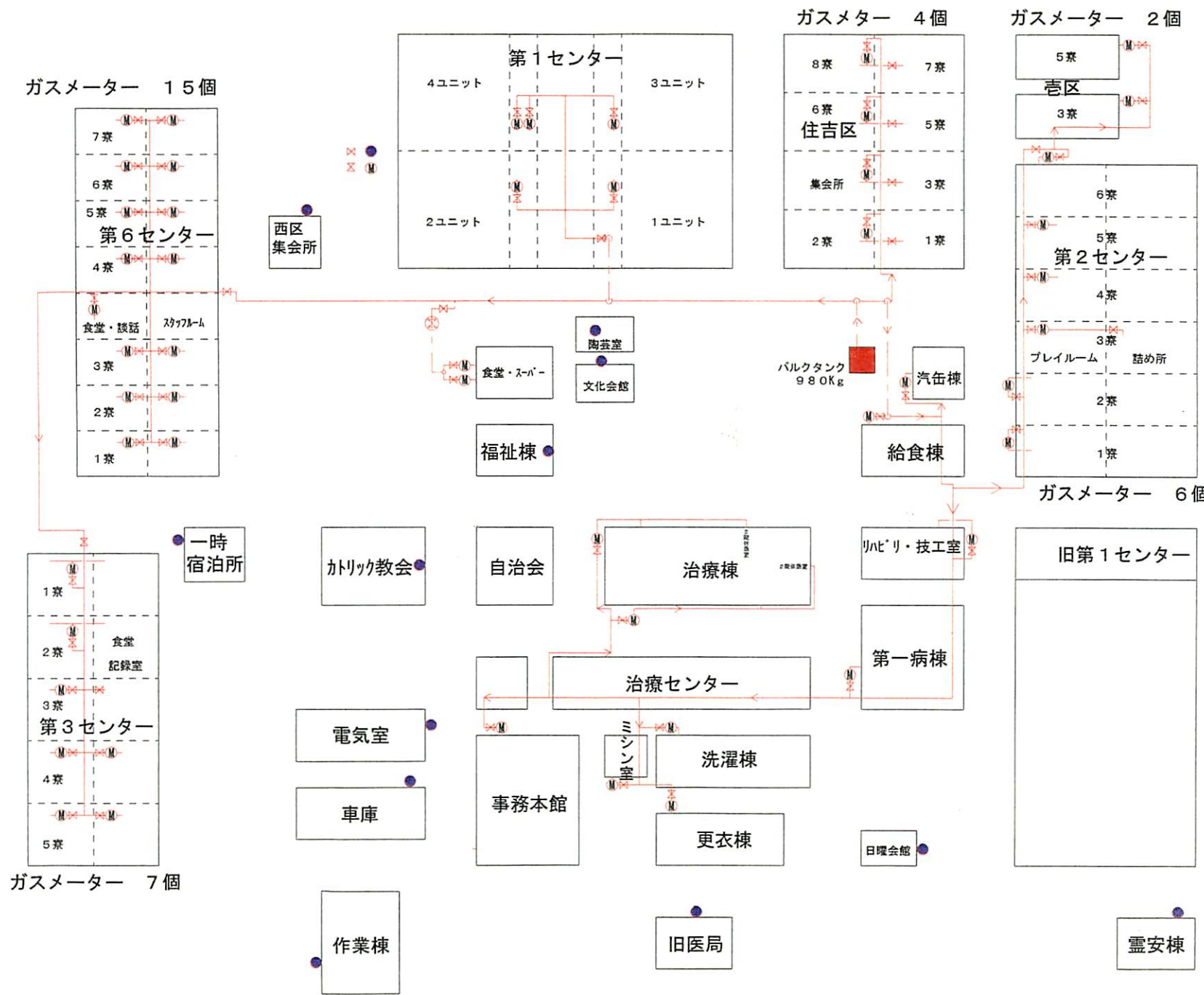
LPガス系統図 H25.4
