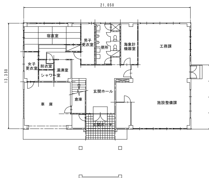
1階平面図
