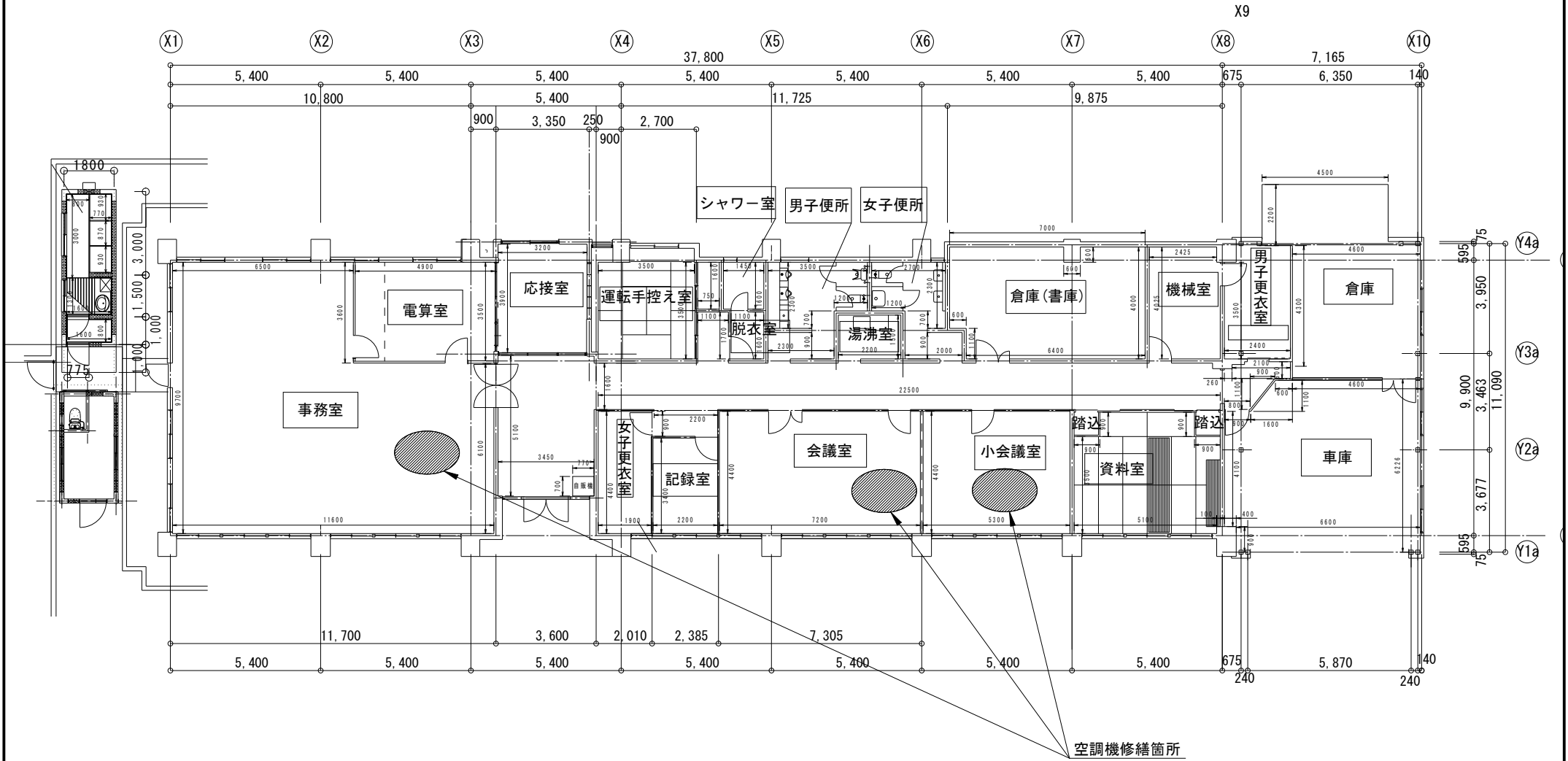
中城湾港出張所平面図
