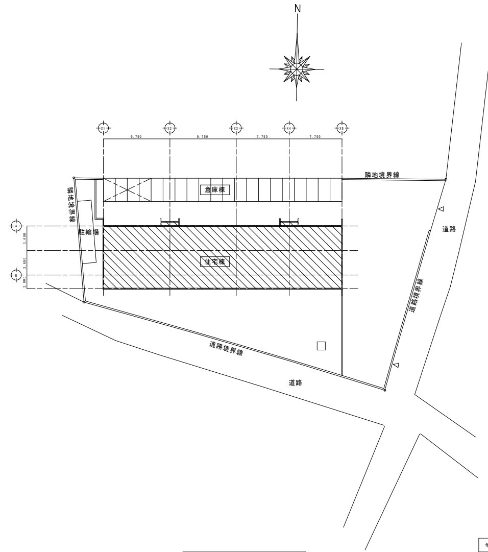
配置図 S=1:400
