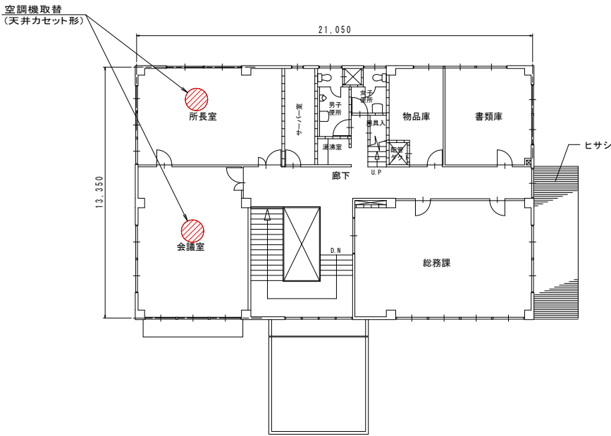
2 階平面図
