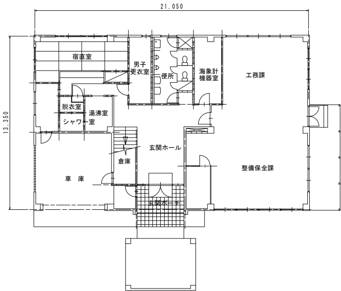
1 階平面図
